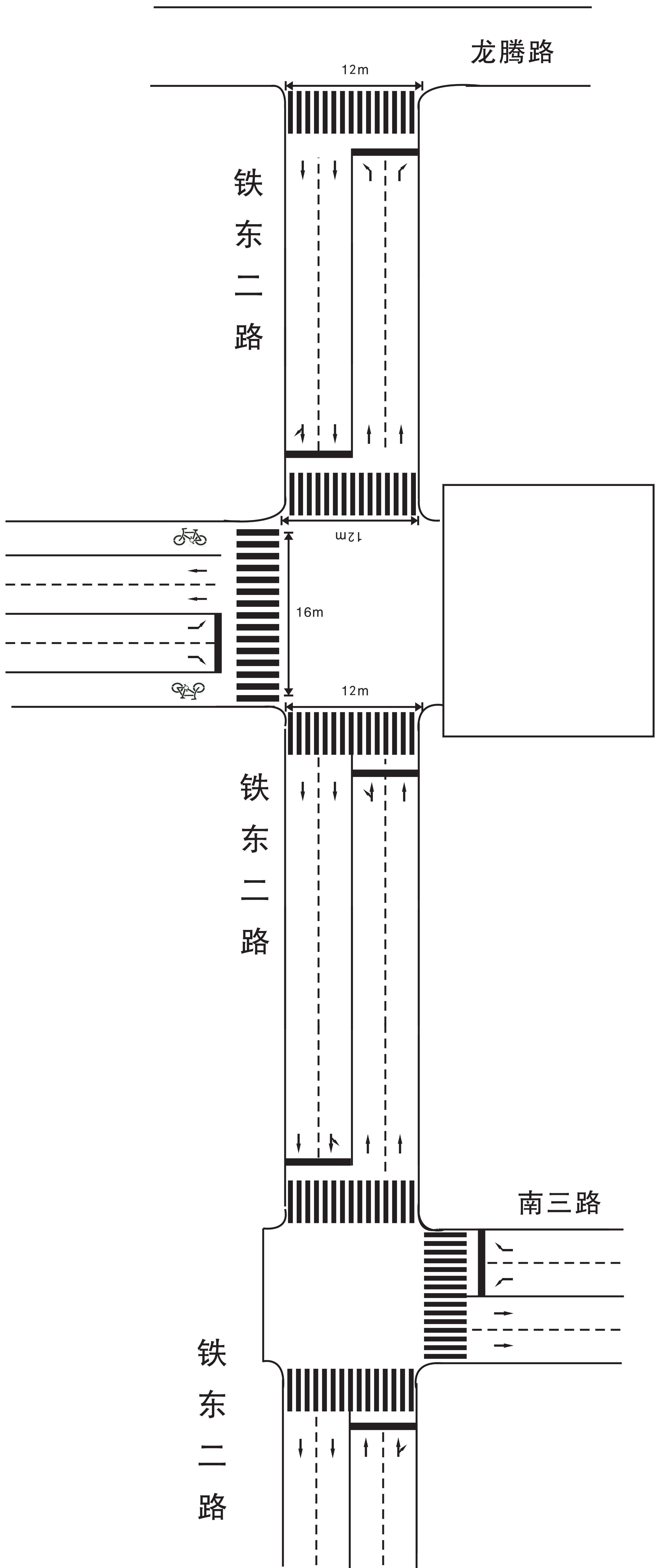
铁东二路 (龙腾路至和平路) 标线标识示意图
