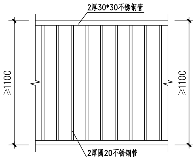
玻璃栏板防护栏杆详图 1:20
